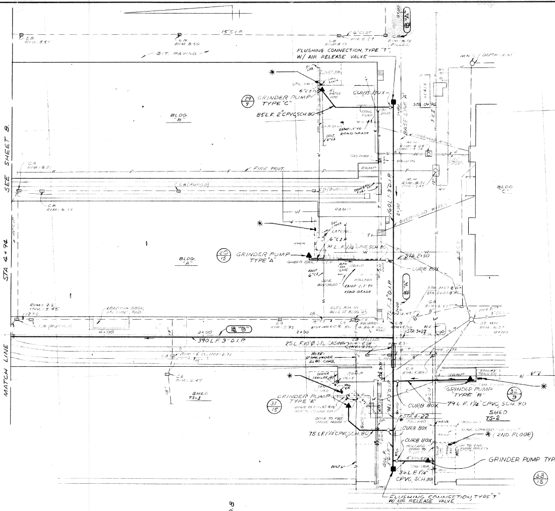
PLAN SCALE: 1" = 30'
